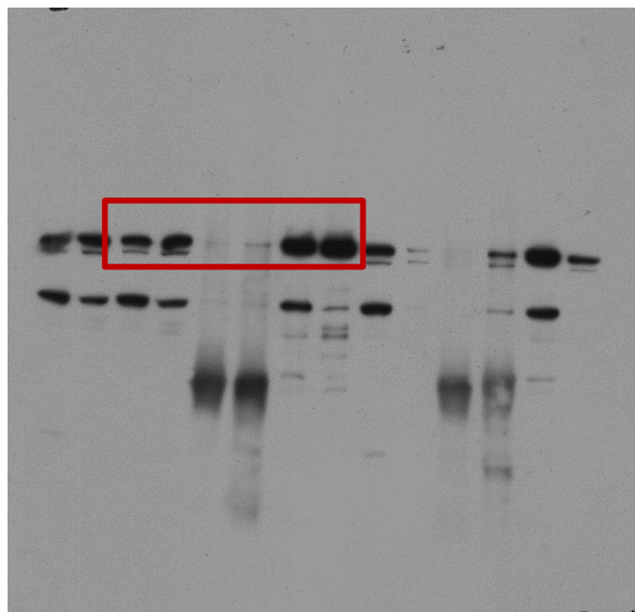
Cdc5
